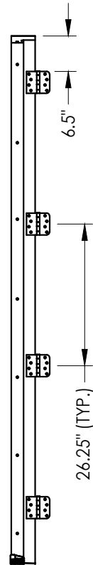
HINGE JAMB
